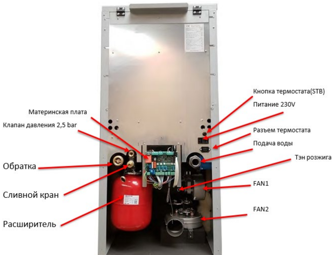
Рисунок 10. Вид сзади на автоматику и основные узлы. Со снятой защитной панелью.
