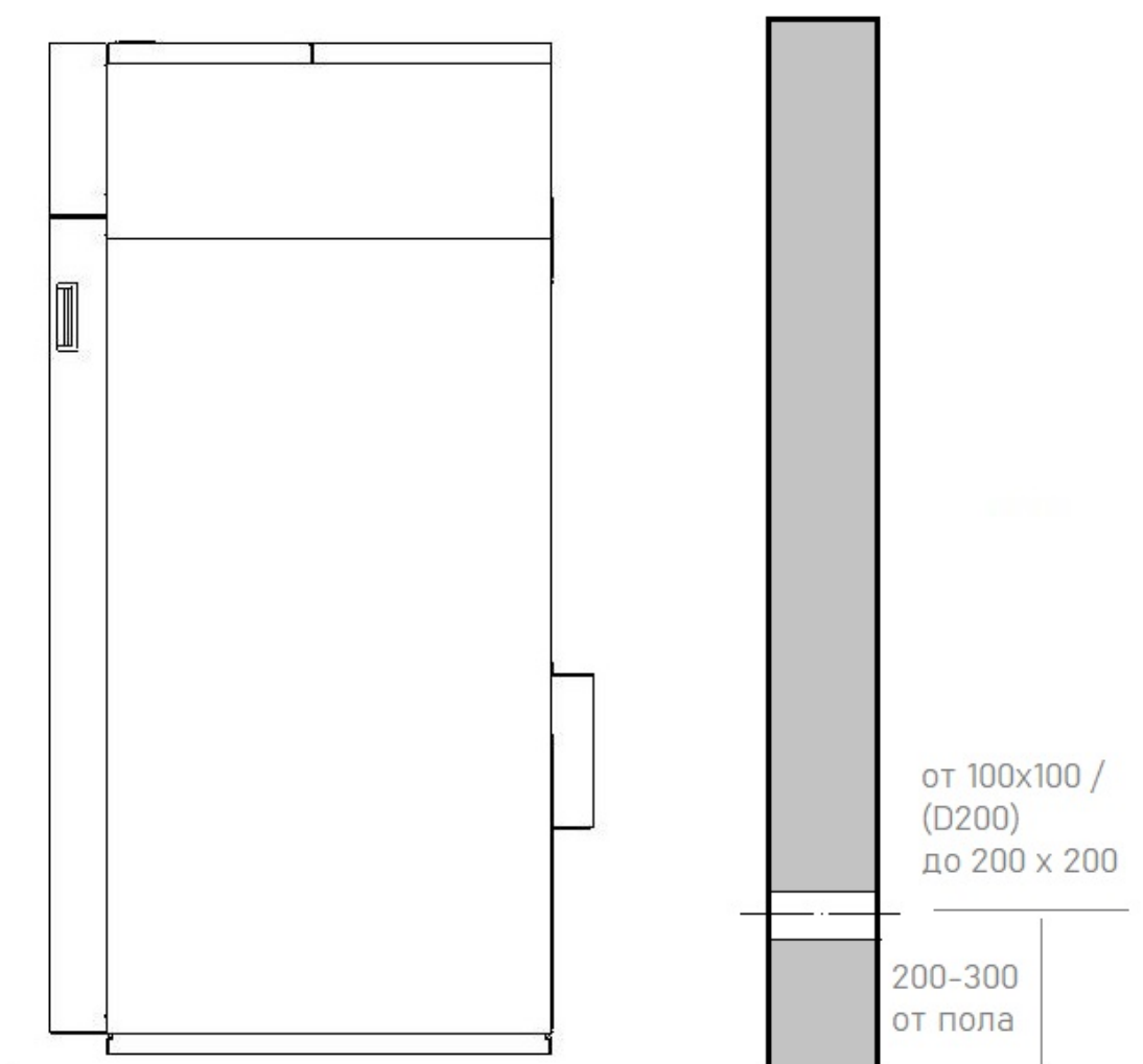
Рисунок 8. Расположение приточного проёма.
