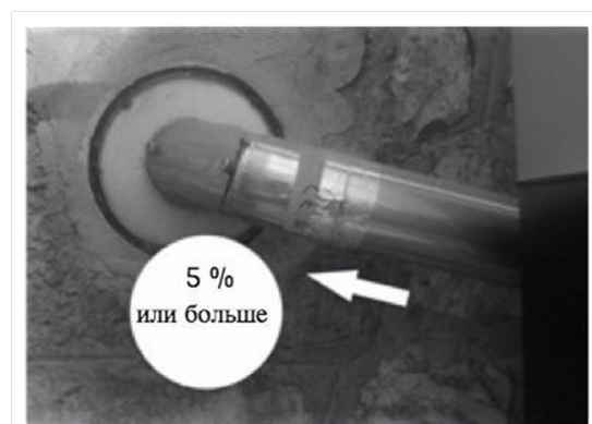
Рисунок 6. Наклон к выходу дымовых газов
