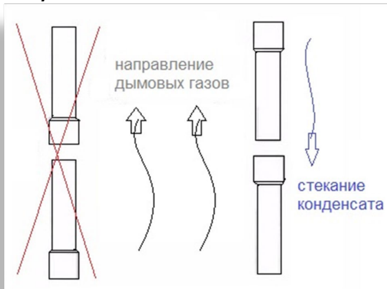
Рисунок 5. Сочленение колен.
